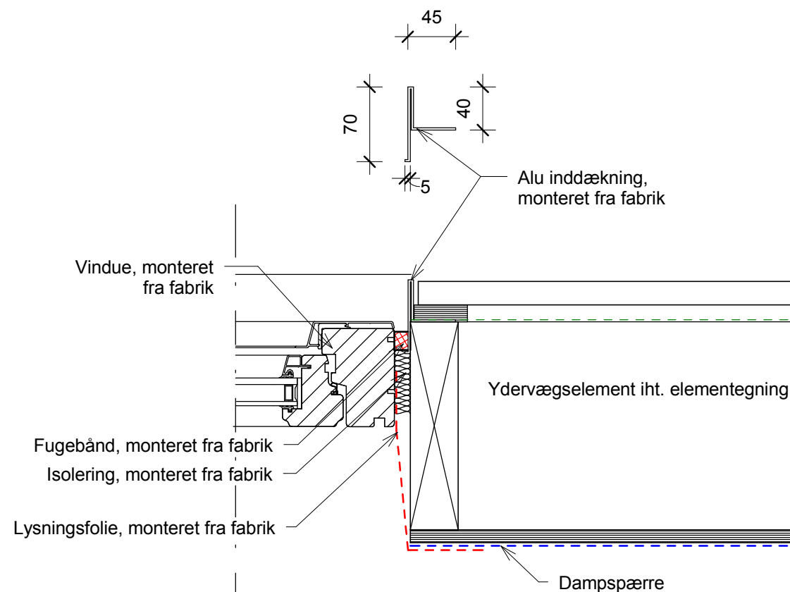
Vandret snit sidekarm
