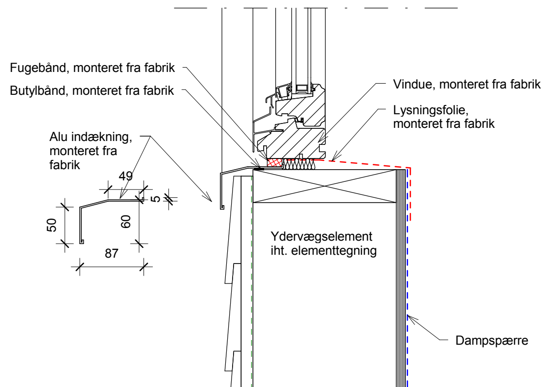
Lodret snit bund- og topkarm
